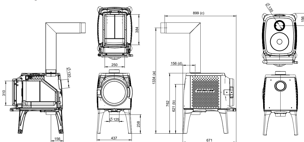
Abb. 2: Abmessungen Grundgerät
