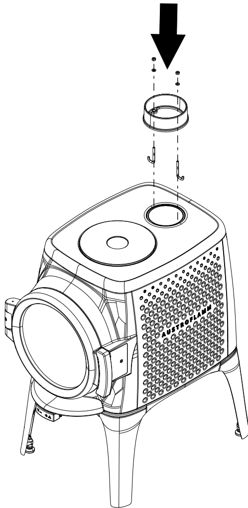
Abb. 7: Rauchrohrstutzen montieren
