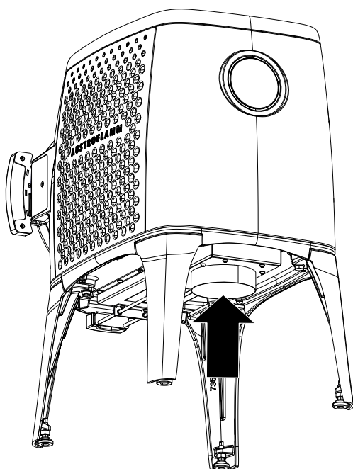
Abb. 10: Aluflexschlauch befestigen
