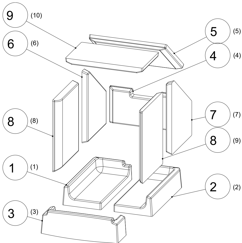
Abb. 11: Keramott
