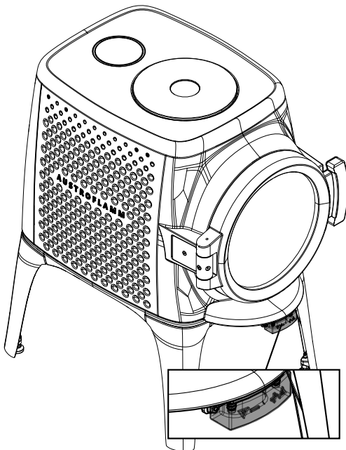
Abb. 13: Primär-Sekundärluftregler
